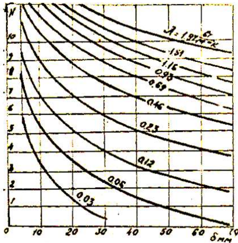
Рис. 2. Диаграмма для выбора ступени мощности нагревательной плиты
