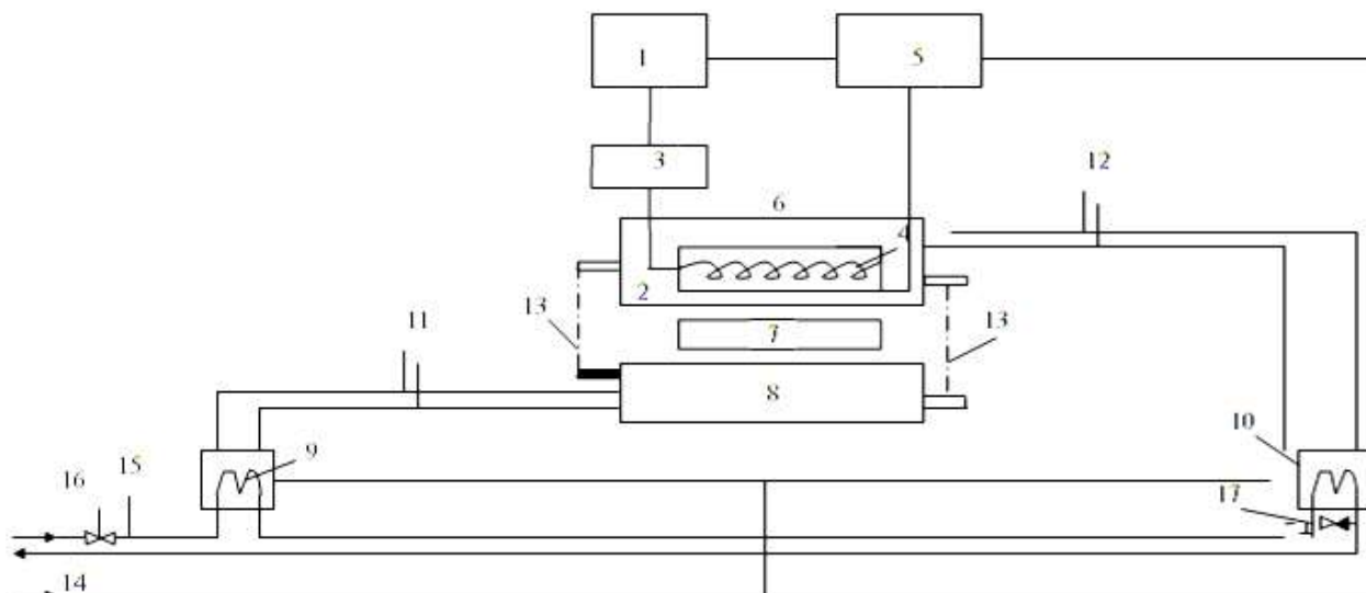
Рис. 1.1. Принципиальная схема установки доктора Бокка:
